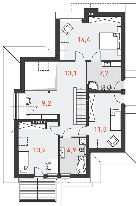
RZUT PODDASZA 80,9 m 2
