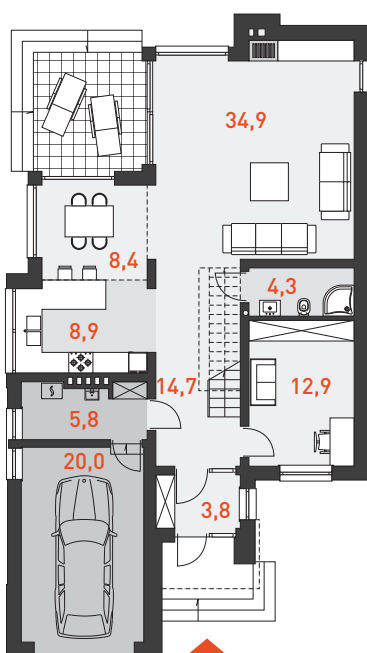
RZUT PARTERU 113,7 m 2
