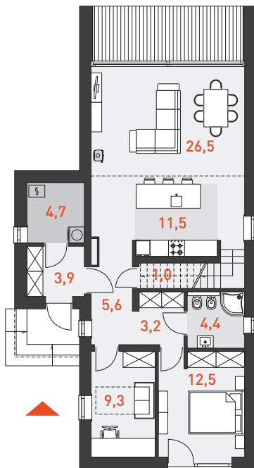
RZUT PARTERU 77,9 m 2
